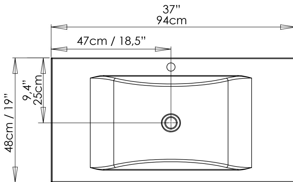
VISTA EN PLANTA / UPPER VIEW
