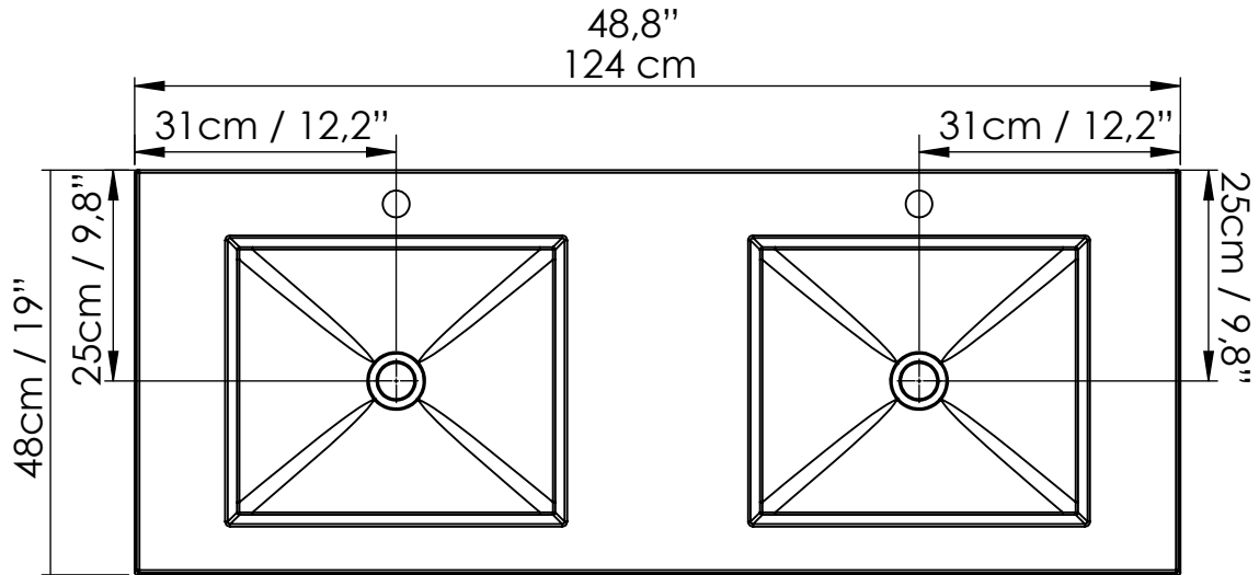
VISTA EN PLANTA / UPPER VIEW
